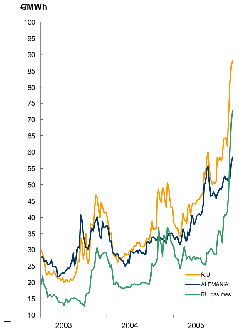
PRECIO DE ENERGÍA ELÉCTRICA Y GAS
