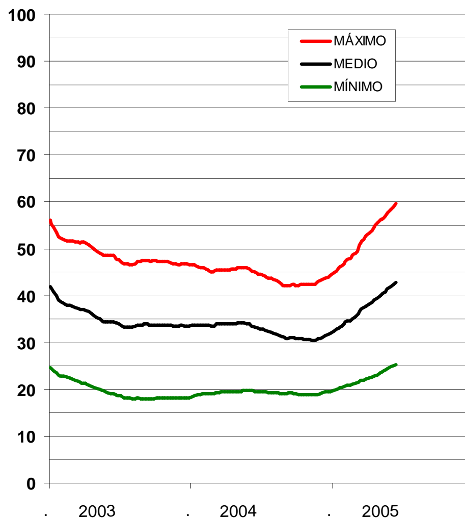
ESPAÑA: PRECIO OMEL FINAL PARA CLIENTE CUALIFICADO €/MWh Datos: Media móvil de 52 semanas
