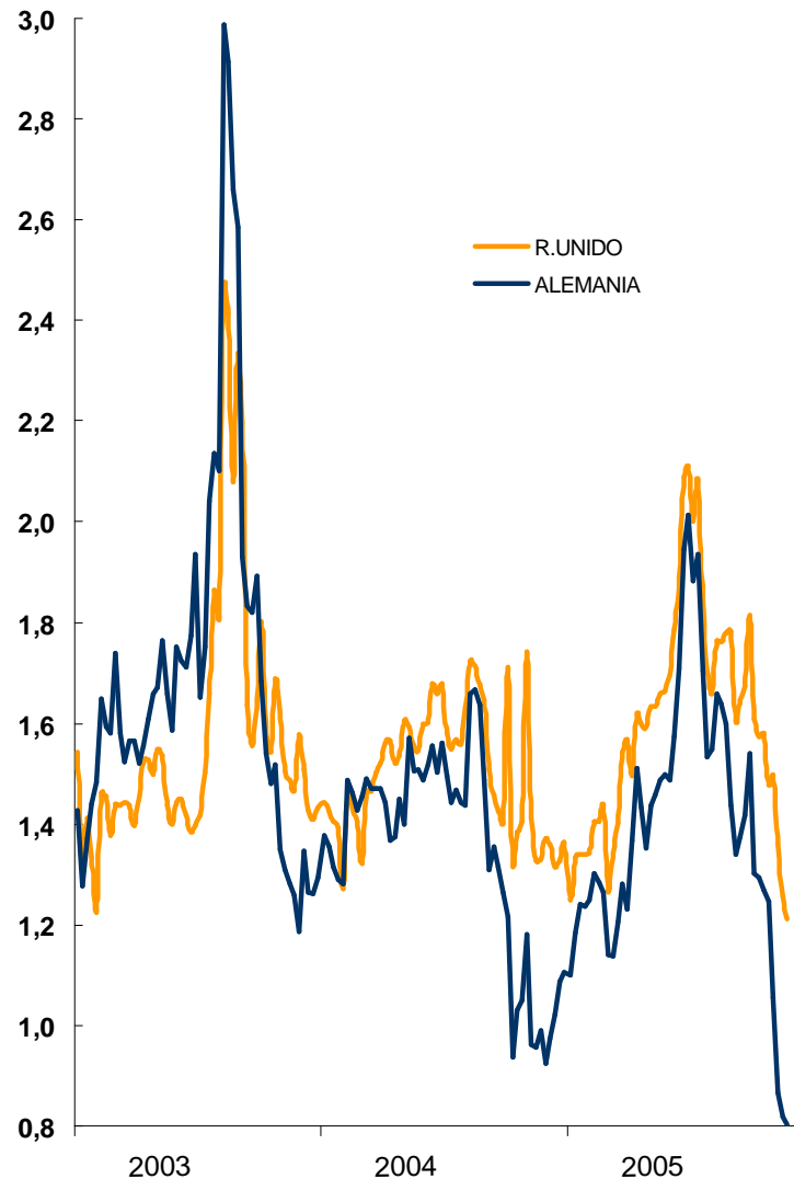
RELACIÓN ENTRE EL PRECIO DE LA ENERGÍA ELÉCTRICA EN EL REINO UNIDO Y ALEMANIA EN RELACIÓN AL PRECIO GAS EN R.UNIDO
